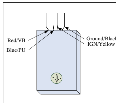
圖示五. 外型圖
