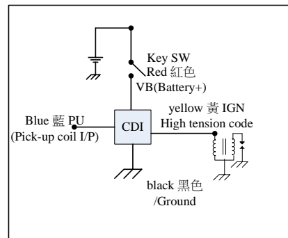
圖示四. 實車配線圖
